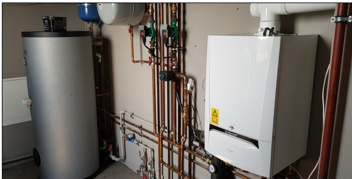
Kocioł gazowy wraz z instalacją
